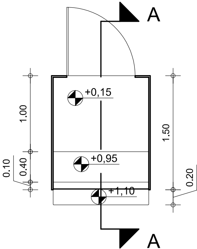
ΚΑΤΟΨΗ
