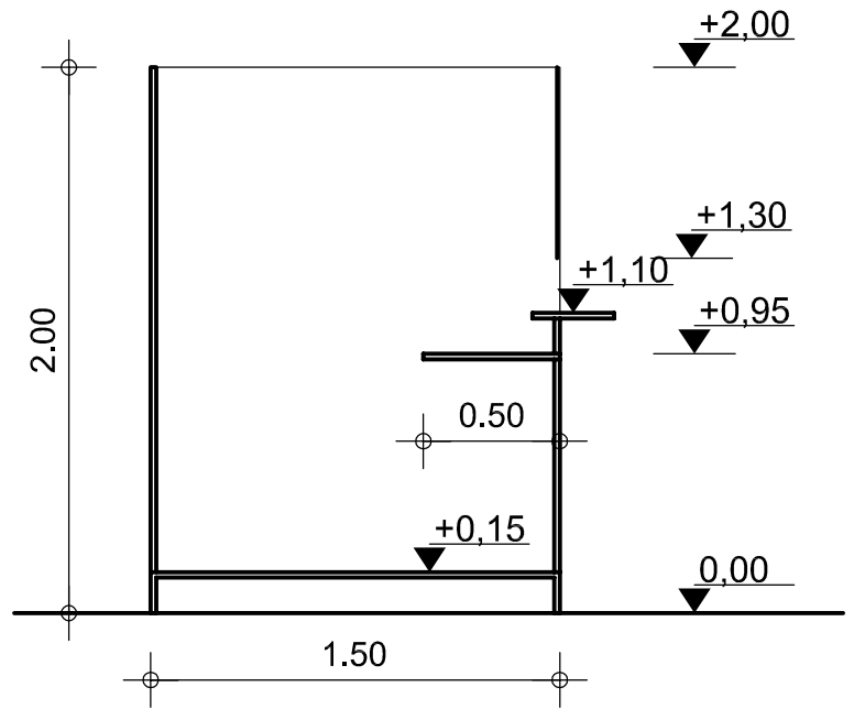
ΤΟΜΗ Α-Α
